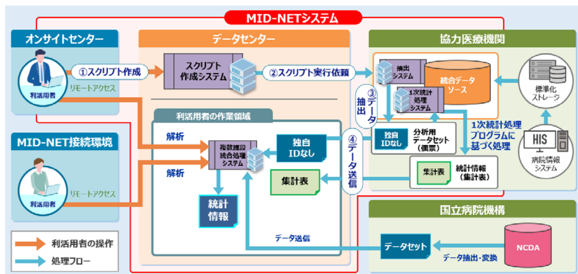
図1 MID-NET システムの概要
